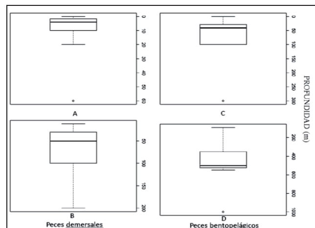
Figura 2: Análisis de cuartiles de las profundidades máximas y mínimas preferidas por las especies actuales representativas de las 10 familias registradas para Fm. Bahía Inglesa. La línea negra representa la mediana de los datos.
